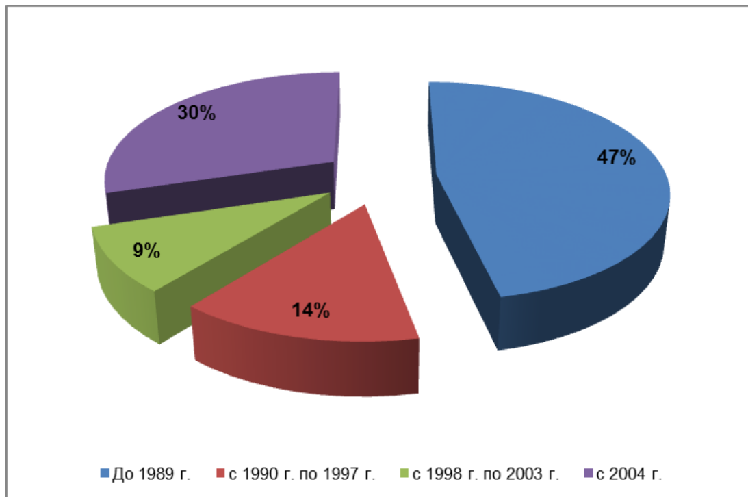
Рисунок 1.4 – Распределение протяженности трубопроводов тепловых сетей ООО «БашРТС» по годам прокладки
