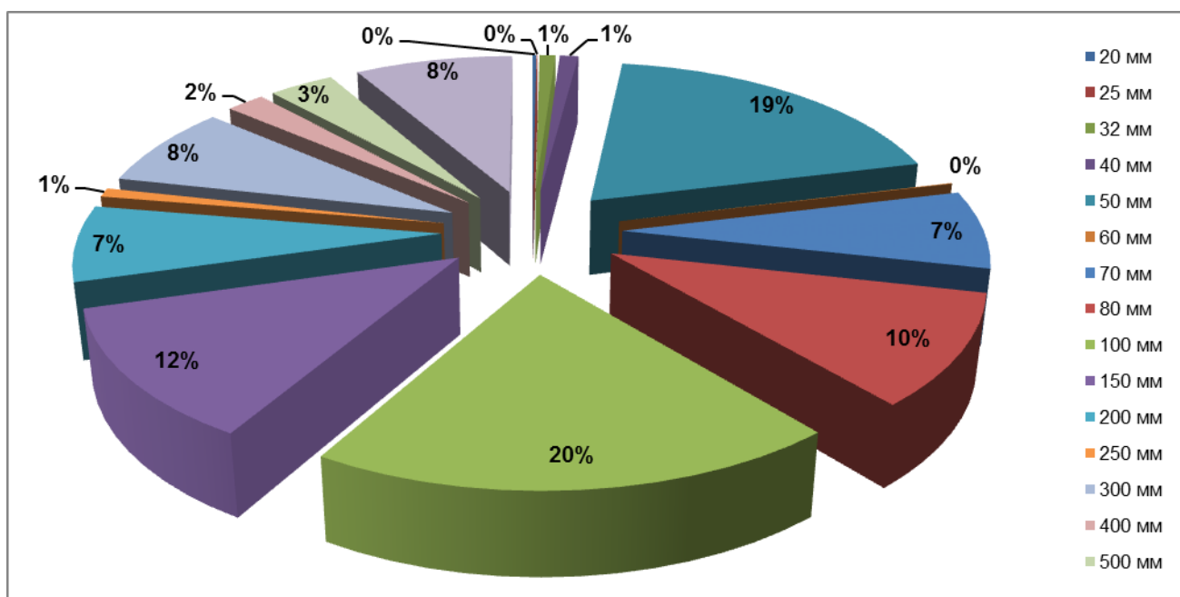
Рисунок 1.2 – Распределение протяженности трубопроводов тепловых сетей ООО «БашПТС» по диаметрам
