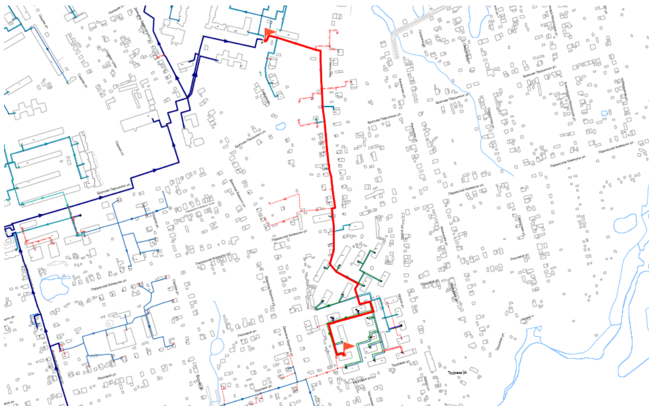
Рисунок 2.7 - Путь теплоносителя по направлению от «ЦТП – 11» до перспективного потребителя «ПП_11»
