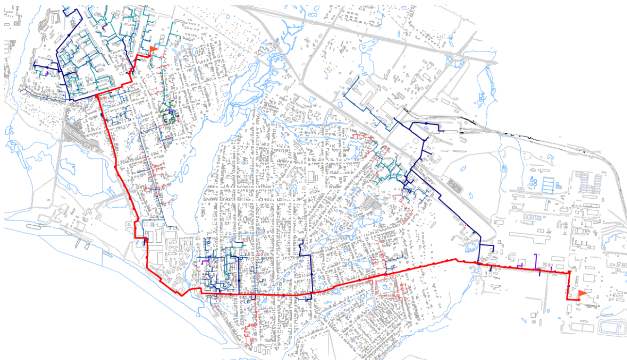
Рисунок 2.5 - Путь теплоносителя по направлению от Приуфимской ТЭЦ до обобщенного потребителя «ЦТП - 11»
