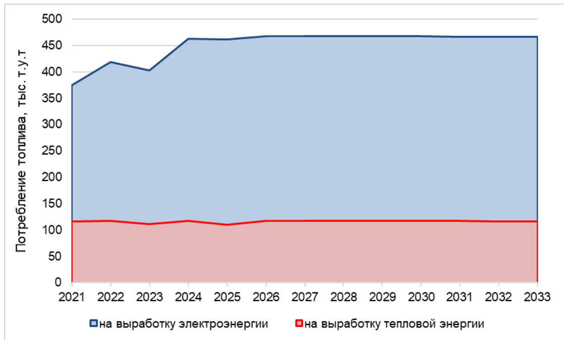
Рисунок 2.1 – Суммарное потребление топлива на выработку тепловой и электрической энергии на Приуфимской ТЭЦ в 2021-2033 годах
