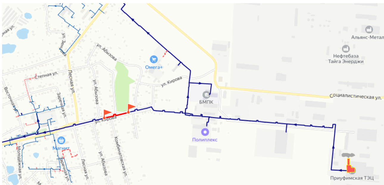
Рисунок 2.1. Отключаемый участок на магистральном тепловом выводе
